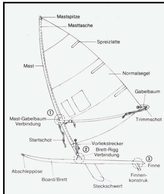
Abb. 1: Das Windsurfgerät (entnommen aus Herreilers & Weichert, 1980).
