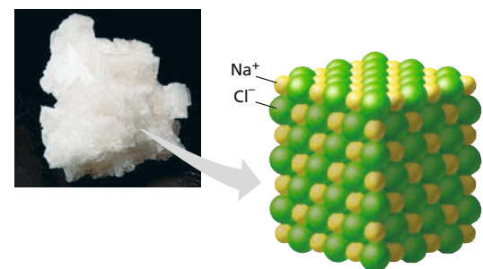
Abbildung 2.9: Ein Kochsalzkristall. Das Natrium-Kation ( Na^+ ) und das Chlorid-Anion ( Cl^- ) werden durch ionische Wechselwirkungen (Ionenbindung) zusammengehalten. Die Summenformel NaCl gibt an, dass das Teilchenverhältnis Na^+ zu Cl^- 1:1 ist.
