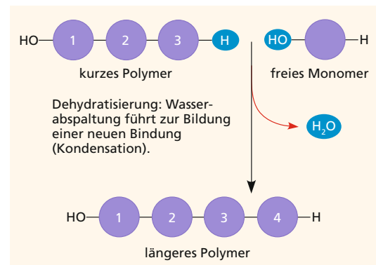
(a) Dehydratisierungsreaktion (Kondensation) bei der Synthese eines Polymers.
