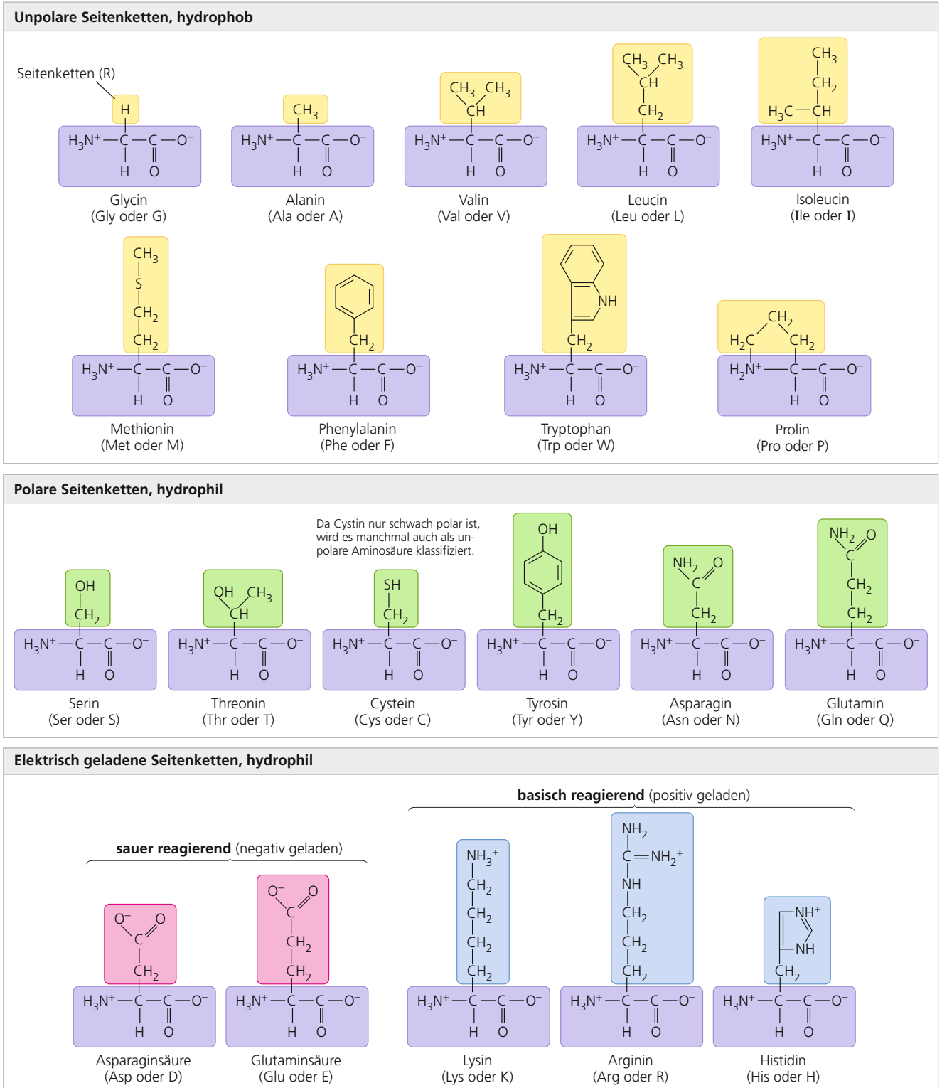
Abbildung 5.13: Die 20 Aminosäuren von Proteinen. In Klammern die Abkürzungen der jeweiligen Aminosäuren im Drei- und im Einbuchstabencode. Die proteinogenen Aminosäuren sind anhand der chemischen Eigenschaften ihrer Seitenketten (R) angeordnet. Alle Aminosäuren sind L-Enantiomere.
