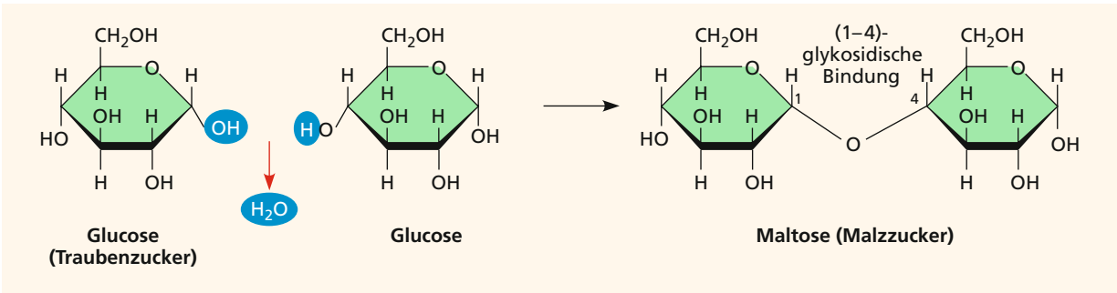
(a) Die Dehydratisierungsreaktion bei der Synthese der Maltose. Bei dieser Glykosidbildung wird das C-1 des einen Glucoserestes mit dem C-4 des zweiten kovalent verknüpft.
