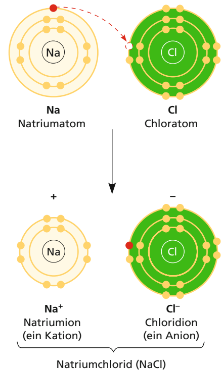
Abbildung 2.8: Elektronenübertragung und Ionenbindung. Eine Ionenbindung wird durch die Anziehung zwischen entgegengesetzt geladenen Ionen (Kationen (+) und Anionen (-)) bewirkt. Sie kann sich auch dann ausbilden, wenn die Ionen nicht zuvor durch eine direkte Elektronenübertragung entstanden sind, sondern Elektronen an andere Partner abgegeben haben.
