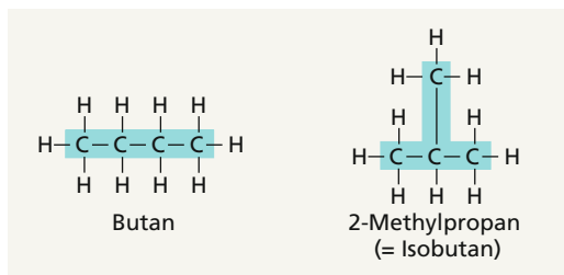
(b) Verzweigungsgrad. Molekülgerüste können unverzweigt oder verzweigt sein.
