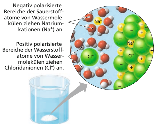
Abbildung 3.4: Die Auflösung von Kochsalz in Wasser. Eine Hülle aus Wassermolekülen umgibt als Hydrathülle jedes gelöste Ion.
