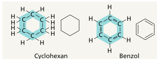
(d) Ringe. In den abstrahierten Strukturformeln (jeweils rechts) symbolisiert jede Ecke ein Kohlenstoffatom (einschließlich der/des daran gebundenen Wasserstoffatome(s)).
