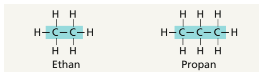
(a) Länge. Kohlenstoffgerüste unterscheiden sich in ihrer Länge.
