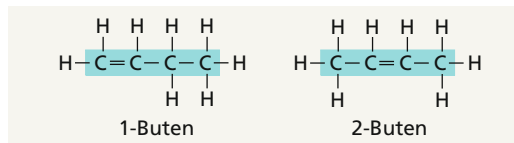
(c) Doppelbindungen. Die Molekülgerüste können Doppelbindungen in variablen Positionen enthalten.
