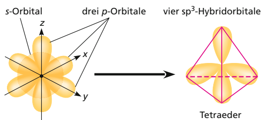
(a) Hybridisierung von Orbitalen bei kovalenten Bindungen. Das einzelne s- und die drei p-Orbitale in der Valenzschale eines Atoms verschmelzen zu vier „tropfenförmigen“ sp^3 -Hybridorbitalen. Diese Hybridorbitale weisen in die vier Ecken eines regelmäßigen Tetraeders (roter Umriss).
