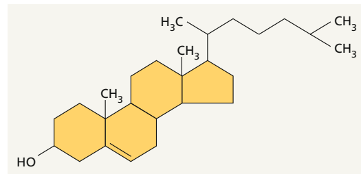
Abbildung 5.12: Cholesterin (Cholesterol), ein Steroid.
