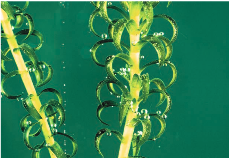
Abbildung 2.12: Photosynthese: die lichtgetriebene Umwandlung von Materie. Elodea sp. (Wasserpest) ist eine in der Aquaristik beliebte Süßwasserpflanze. Sie erzeugt Zucker, indem sie Kohlendioxid- und Wassermoleküle durch die lichtgetriebene Photosynthese umwandelt. Ein großer Teil des so erzeugten Zuckers kann dann in andere Bestandteile der Pflanze überführt werden. Gasförmiger Sauerstoff ( \text{O}_2 ) ist ein Abfallprodukt der Photosynthesereaktion. Auf dem Foto sind die aufsteigenden Blasen des aus den Blättern austretenden Sauerstoffs gut zu erkennen.
