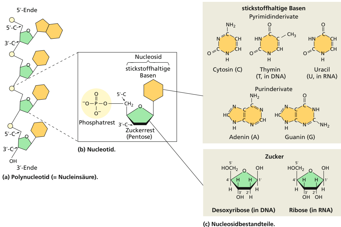
Abbildung 5.18: Bestandteile von Nucleinsäuremolekülen. (a) Polynucleotide bestehen aus einer Zucker-Phosphat-Kette und stickstoffhaltigen Nucleinbasen, die an die Zuckerreste des Polynucleotidrückgrats gebunden sind. (b) Ein einzelnes Nucleotid enthält eine Nucleinbase, die an einen Zucker gebunden ist, und einen Phosphatrest. Das Molekül aus Base und Zucker heißt Nucleosid. (c) Ein Nucleosid besteht aus einer stickstoffhaltigen Nucleinbase (einem Purin- oder Pyrimidinderivat) und einer Pentose (Desoxyribose oder Ribose).
