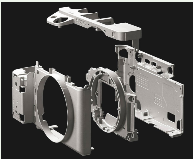
▼ Abbildung 1.11 Bauteile aus Magnesiumlegierung der α6300 (Bild: Sony)
