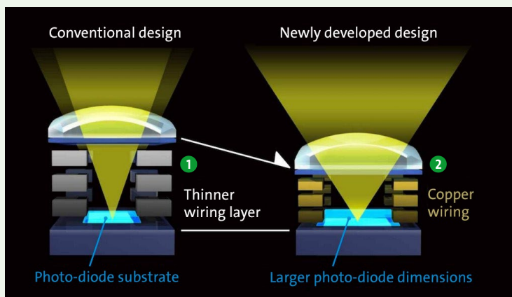
▲ Abbildung 1.12 Gegenüber einem konventionellen Sensoraufbau ① mit kleineren Fotodioden sind die Sensorpixel der \alpha 6300 dünner aufgebaut ②, haben eine Kupferverdrahtung und größere lichtempfindliche Fotodioden (Bild: Sony).
