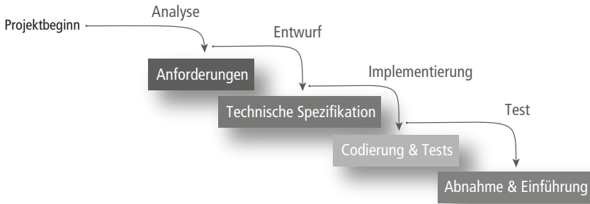
Abbildung 1: Das Wasserfall-Modell
