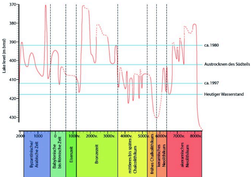
Abb. 2: Rekonstruktion des Wasserstands des Toten Meeres auf Grund von Bohrkernen, die dort entnommen wurden. Der Wasserstand fiel von der Bronzezeit zur Eisenzeit enorm (copyright: W. Zwickel).
