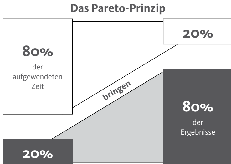
Abb. 9: Das Pareto-Prinzip
