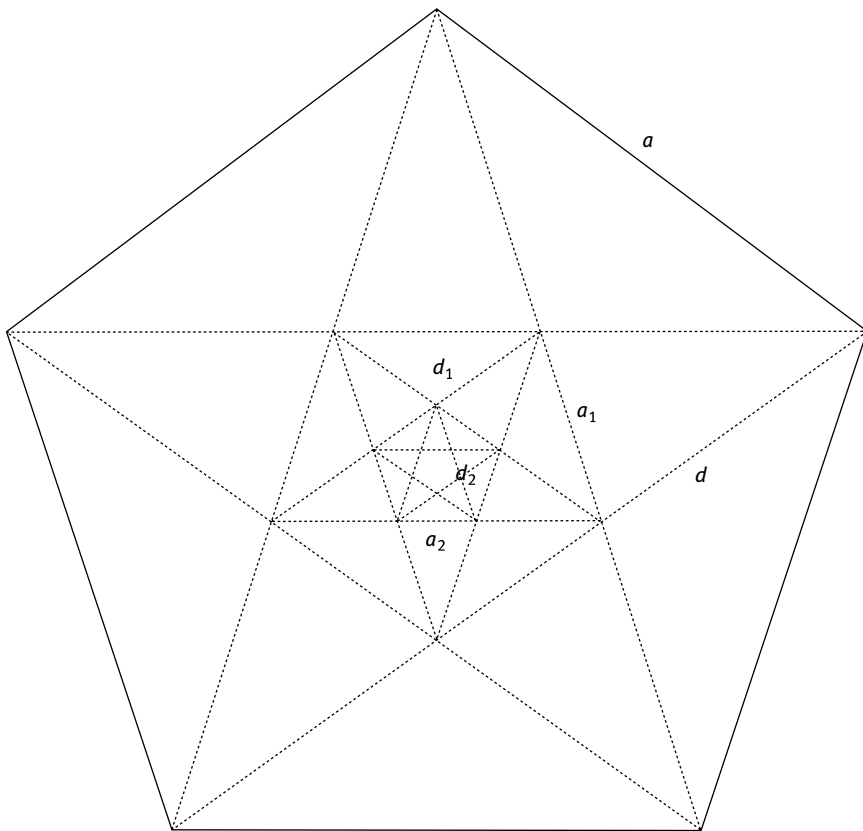
Abbildung: Anfang einer unendlichen Folge regelmäßiger Fünfecke.
